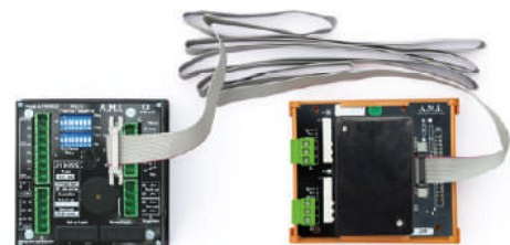
DIN-Platine M0901 „Übertragungsrelais“, angeschlossen an Tafel J1905S
